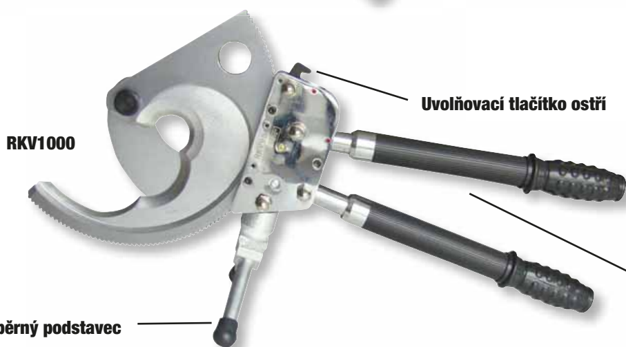
Teleskopická rukojeť
