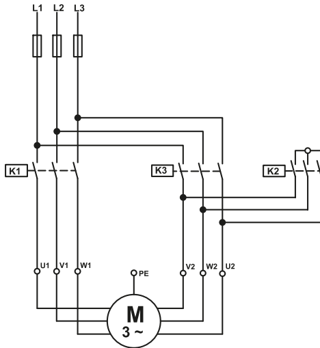
Hauptstromkreis
