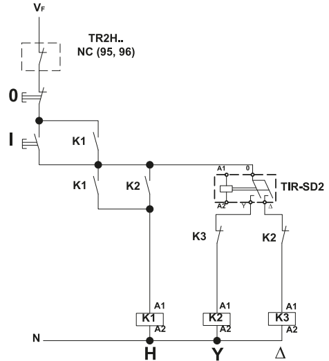
Steuerstromkreis
