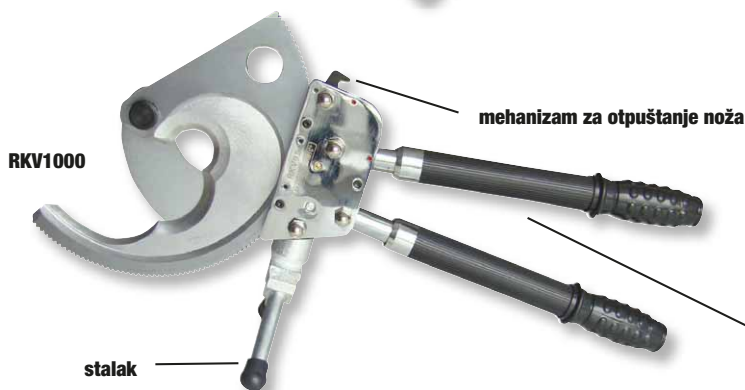
teleskopska ručka
